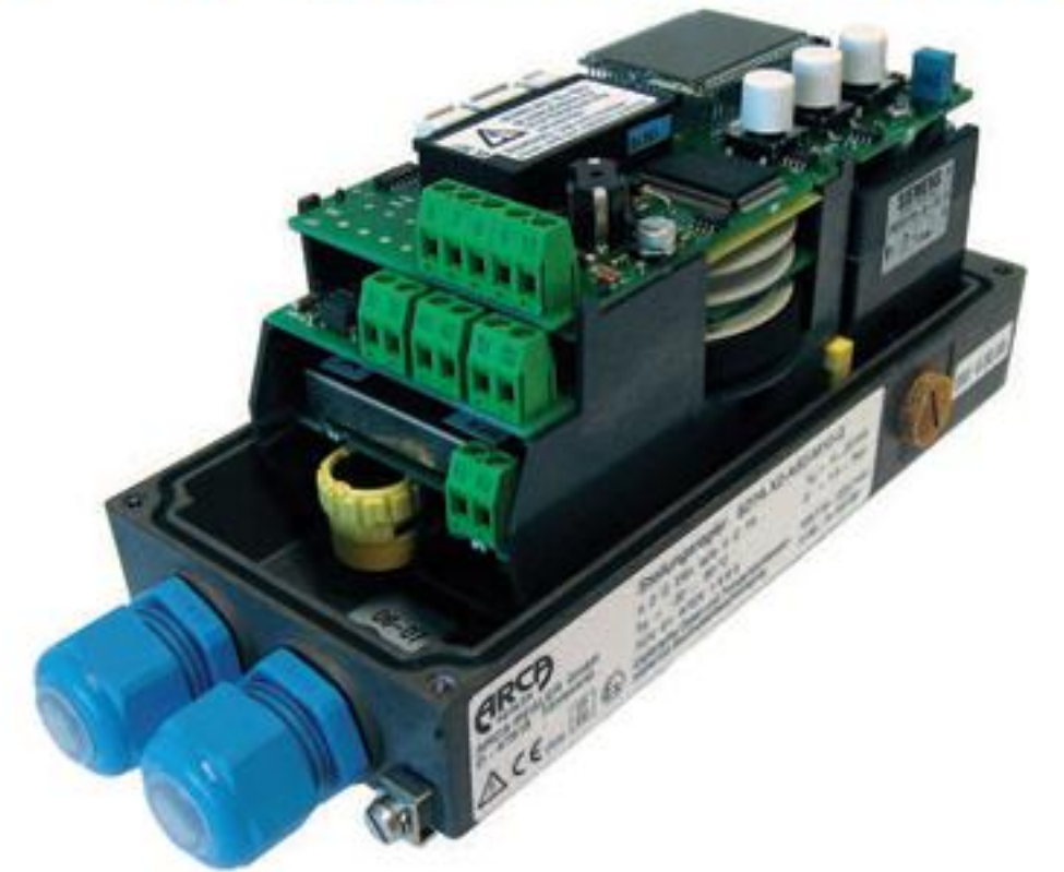
Positioner ARCAPRO OPOS interface
