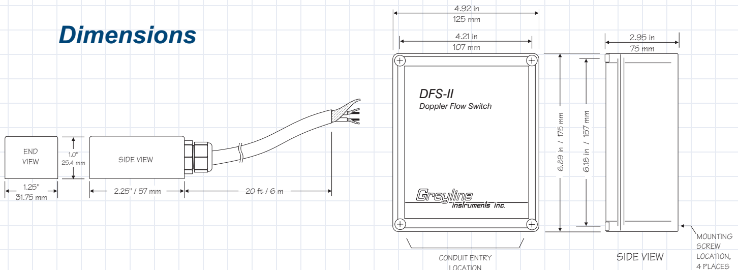
SE3 DOPPLER SENSOR
